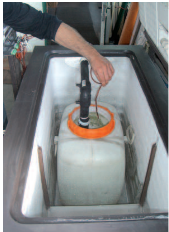
Abb. 4 Fluidbehälter in der Frostbox mit MEG
