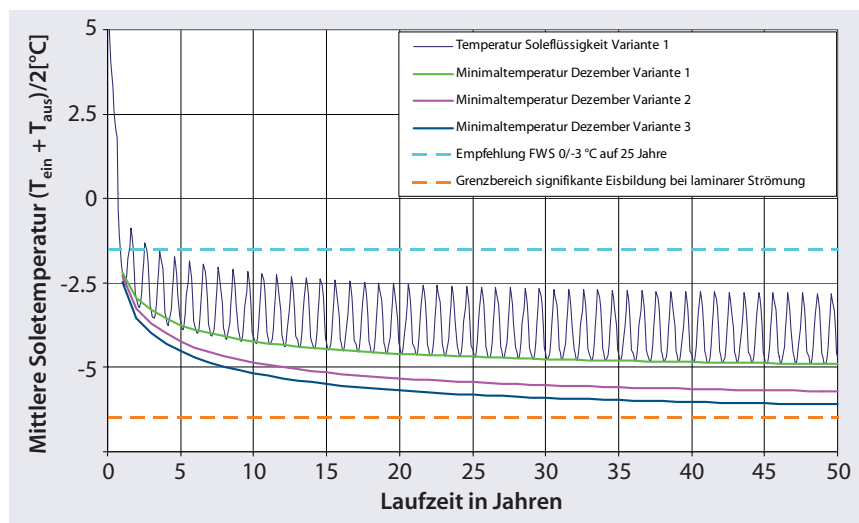
▷ Abb. 2 Simulierter Temperaturverlauf (Mittel der Sole aus Vor- und Rücklauf) des Ist-Zustandes für die EWS im EFH über einen Zeitraum von 25 Jahren, Rote Linie = Grenzwert für Eisbildung (aus [6])
