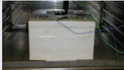
Abb. 9 Mess- und Prüfanordnung im automatischen Klimaschrank
